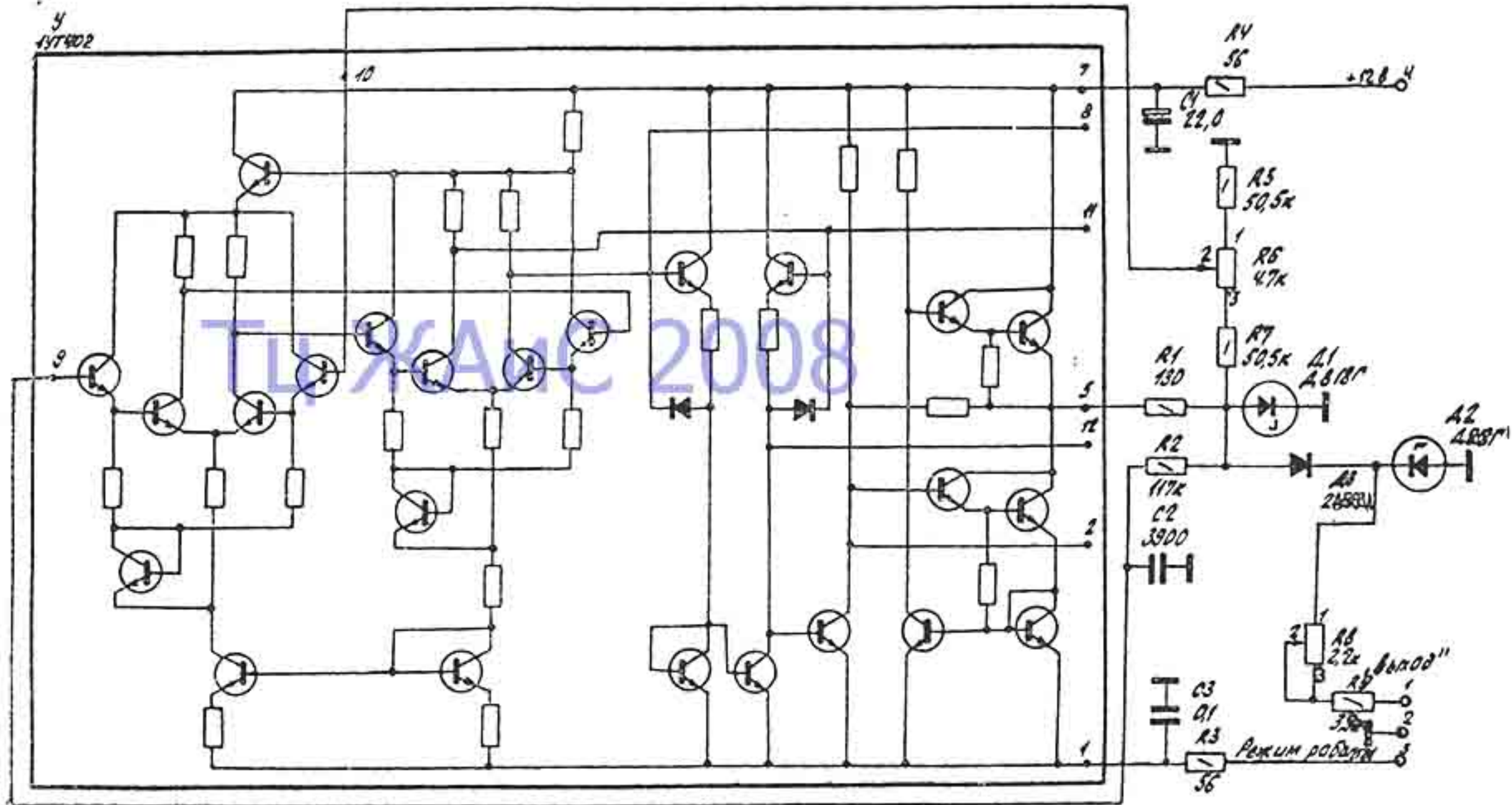
Осциллограф универсальный С1-79 Калибратор
